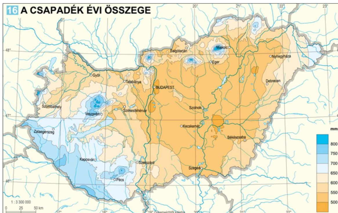
24. ábra: A csapadék évi összege Magyarországon (mm)
