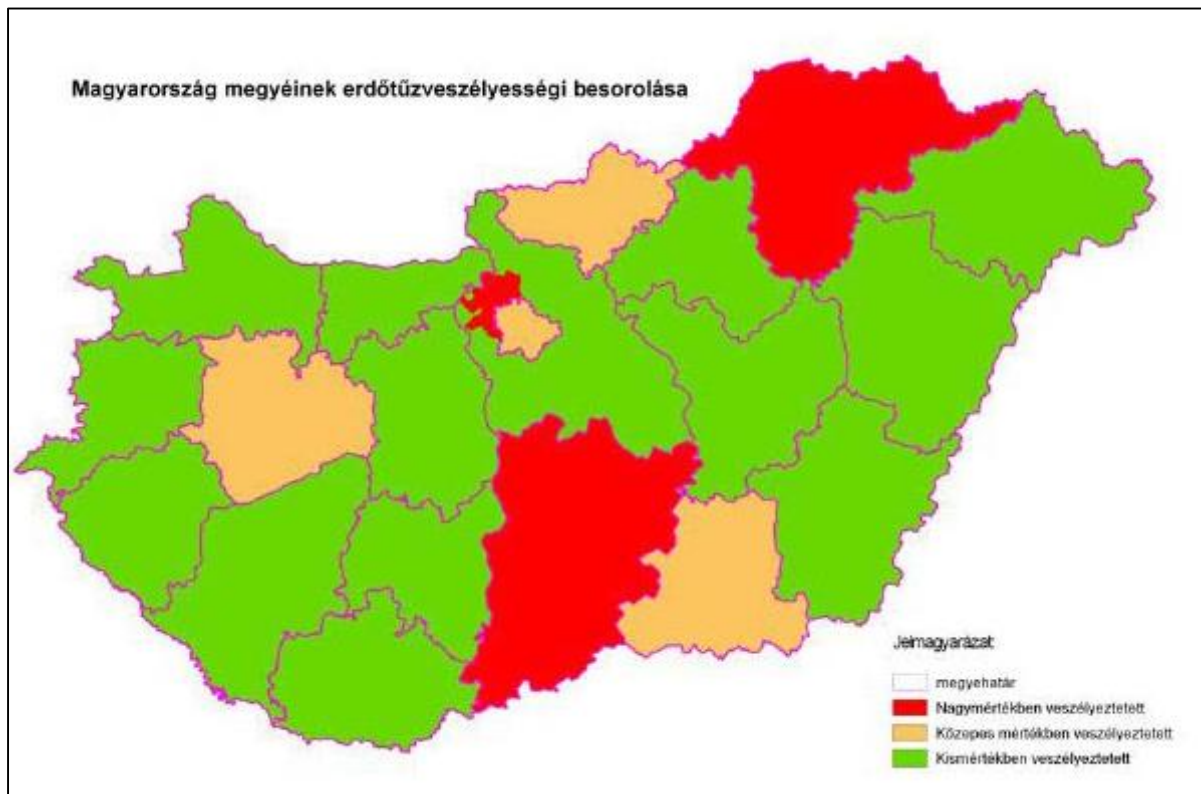
42. ábra: Magyarország megyéinek erdőtüz veszélyességi besorolása 122
